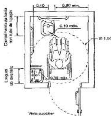
Figura 1 - Detalhe típico de banheiro PNE
