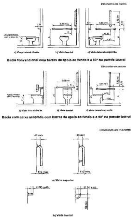
Figura 2 - Detalhe bacias e barras de apoio.
